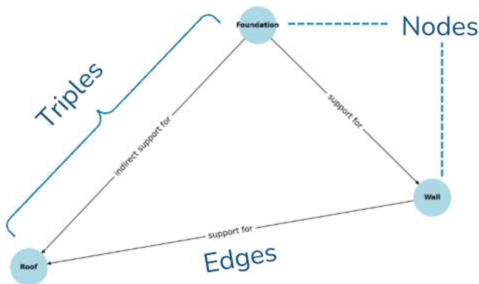
Рис. 6.1-7 Модель данных RDF: узлы (Nodes), связи (Edges) и тройки (Triples), иллюстрирующие отношения между строительными элементами.
