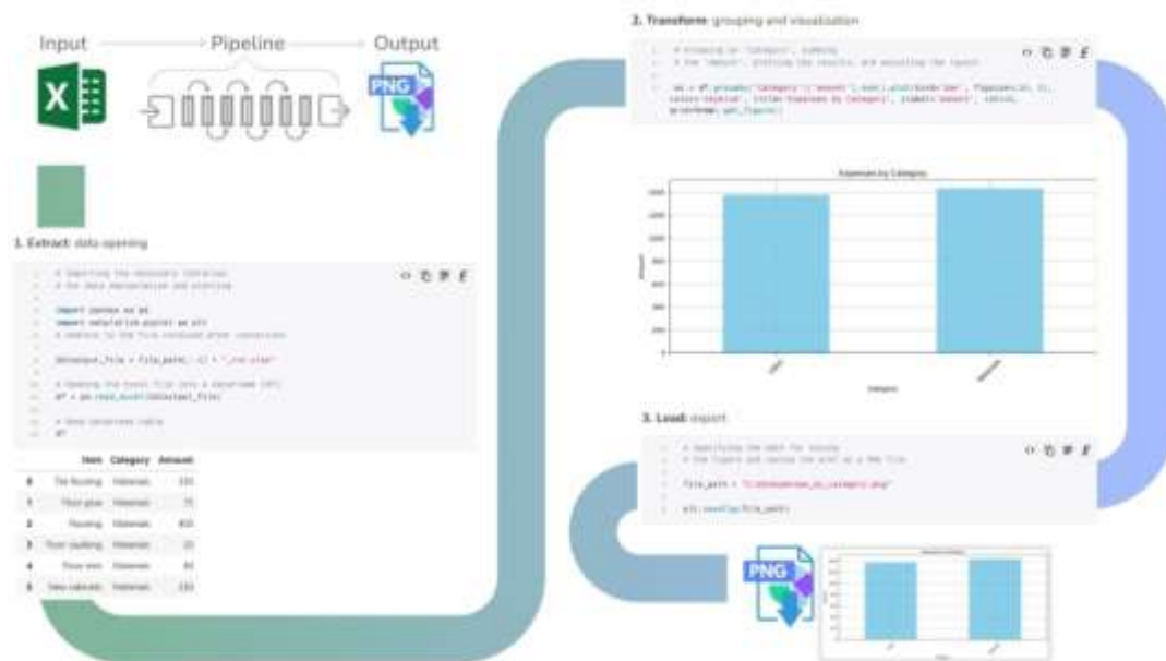
Рис. 7.3-3 Пример ETL Pipeline по автоматическому получению графика из табличных данных в файле XLSX без открытия Excel.
