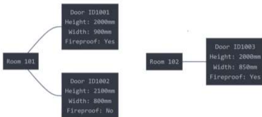
Рис. 3.2-9 Информация о сущностях дверей проекта в графовом представлении.
