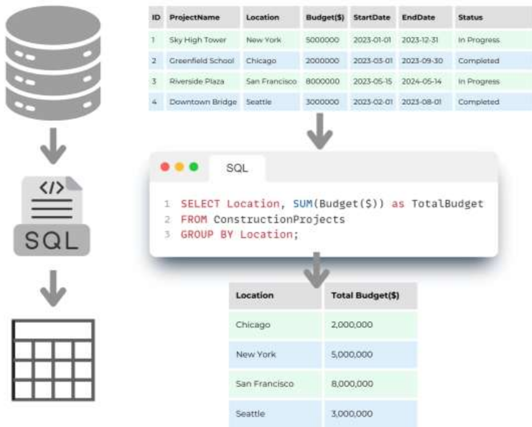
Рис. 3.1-7 Пример DML в SQL: быстрая обработка, группировка и агрегирование при помощи нескольких строк кода для автоматической обработки данных.
